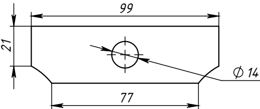
Поз.4 (Ушко) развертка
