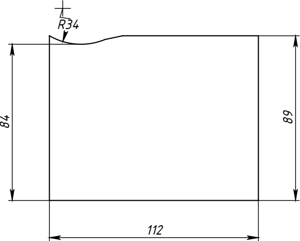
Поз.2 (Угольник) развертка
