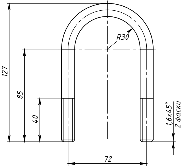
Поз.5 (Хомут)
